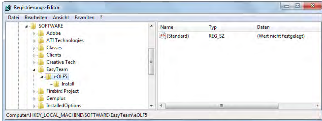
Abbildung 53: EasyTeam-Schlüssel in der Windows Registrierung
