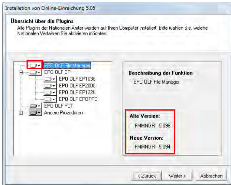
Abbildung 38: Vergleich der alten und neuen Version des EPO OLF File Managers
