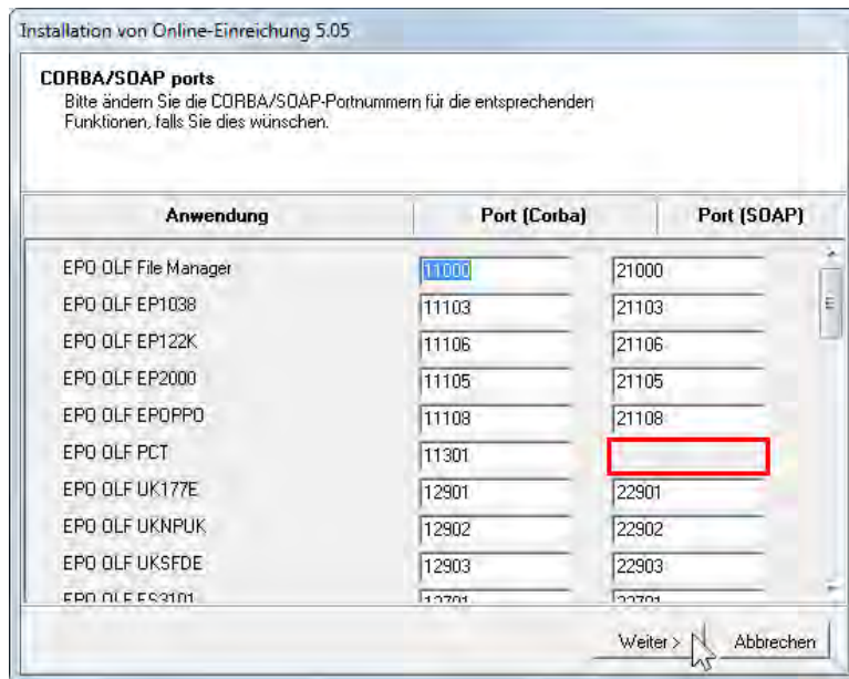
Abbildung 15: Ports für Kommunikation über CORBA und SOAP
