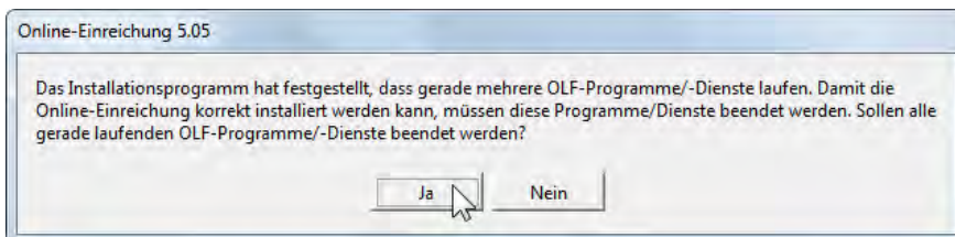
Abbildung 33: Vorgängerversion gefunden
